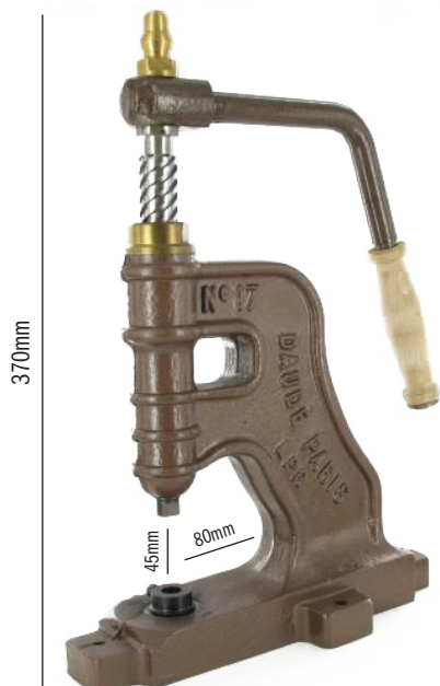
MACHINE N° 17
